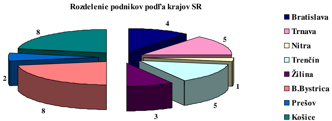
graf č. 1
