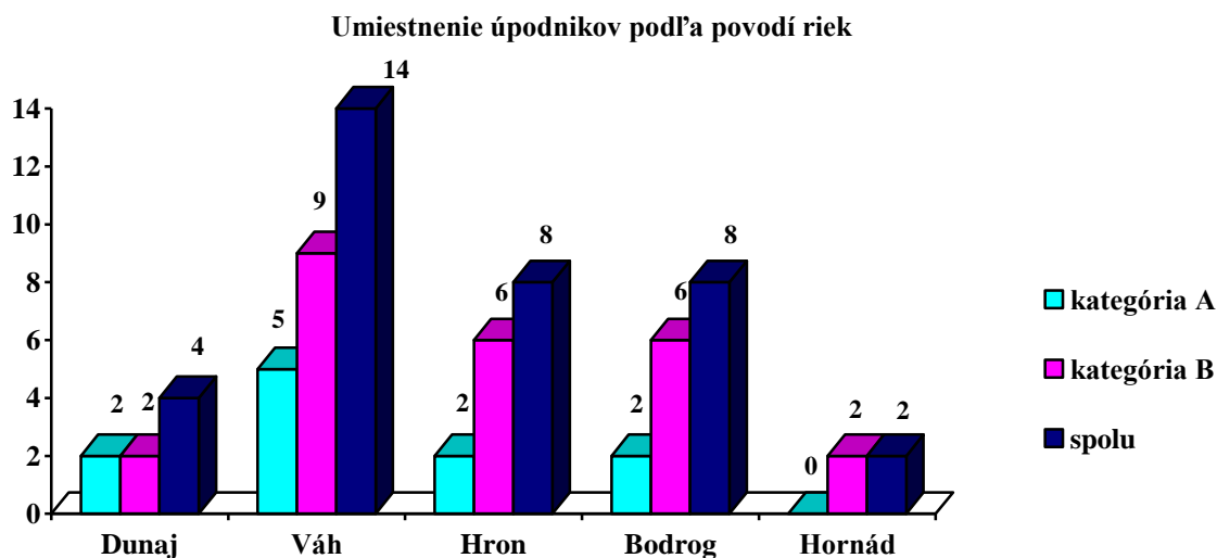
graf č.3
