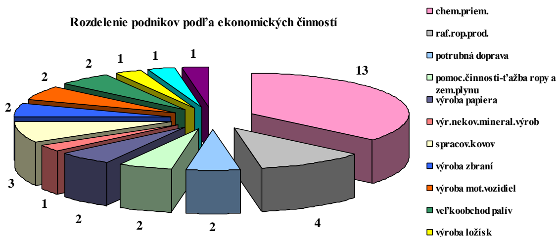
graf č. 4
