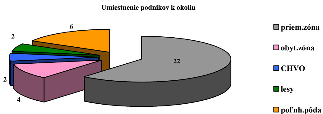
graf č. 2
